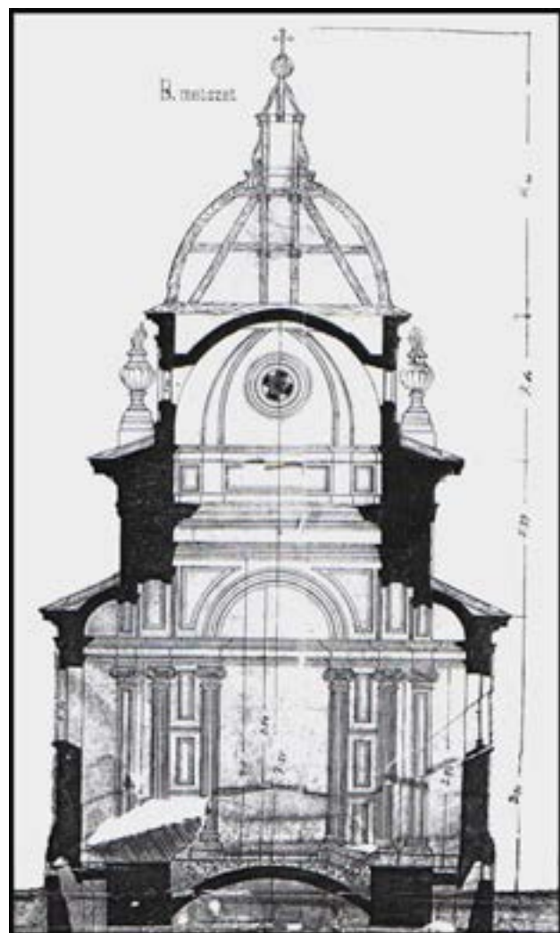
A kápolna terve, metszet
